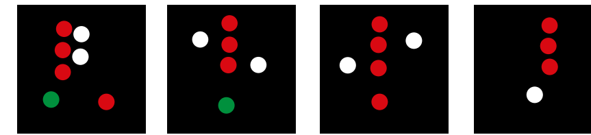
Bugansicht Steuerbordansicht Backbordansicht Heckansicht
