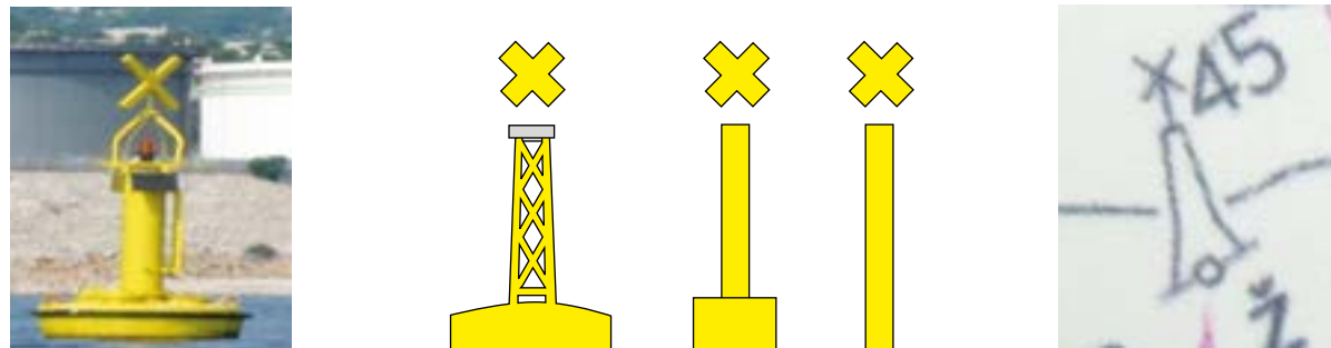
Dieses sind meistens ‚neue Gefahren‘, die noch nicht in den nautischen Warnungen veröffentlicht wurden. Sie können aber auch für besondere Gebiete und Stellen, wie beispielsweise Warngelände oder -stellen, Fischereigründe, Baggerschüttstellen, Kabel oder Rohrleitungen stehen. Die Tonne ist gelb mit einem X am Topp.
