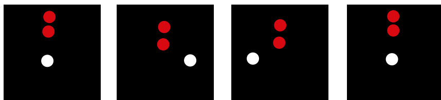
Bugansicht Steuerbordansicht Backbordansicht Heckansicht
